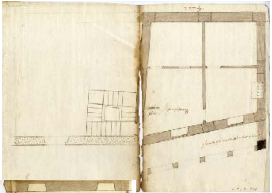
Plano Planta primera (AHPZA, Fondo MPyD, 3/2)
